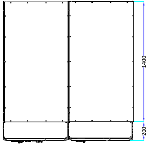
ÜST GÖRÜNÜM TOP VIEW
