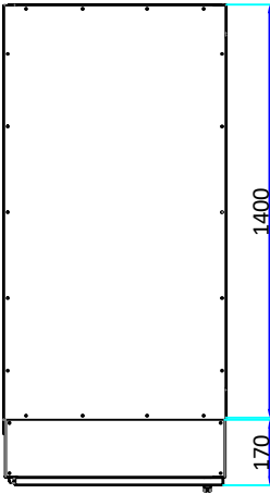
ÜST YÜZ TOP VIEW
