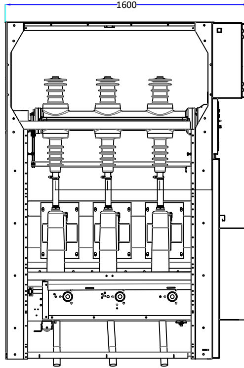
YAN GÖRÜNÜM RIGHT VIEW
