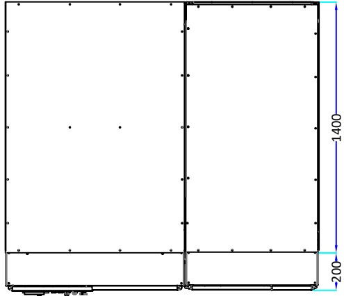
ÜST GÖRÜNÜM TOP VIEW
